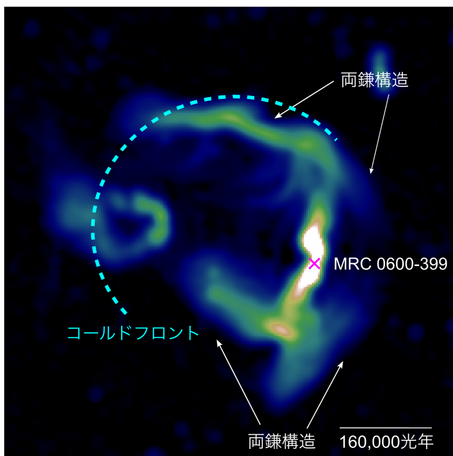
図 2: 電波干渉計ミーアキャットで観測された銀河 MRC 0600-399 のジェットの姿。X印のところにブラックホールが存在し、そこから上下にジェットが吹き出している。上下に吹き
